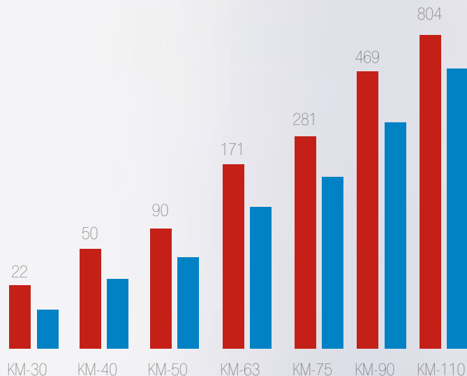
■ GAMME KM CIDEPA SINCRON (Couple Nm) ■ AUTRES FABRICANTS
